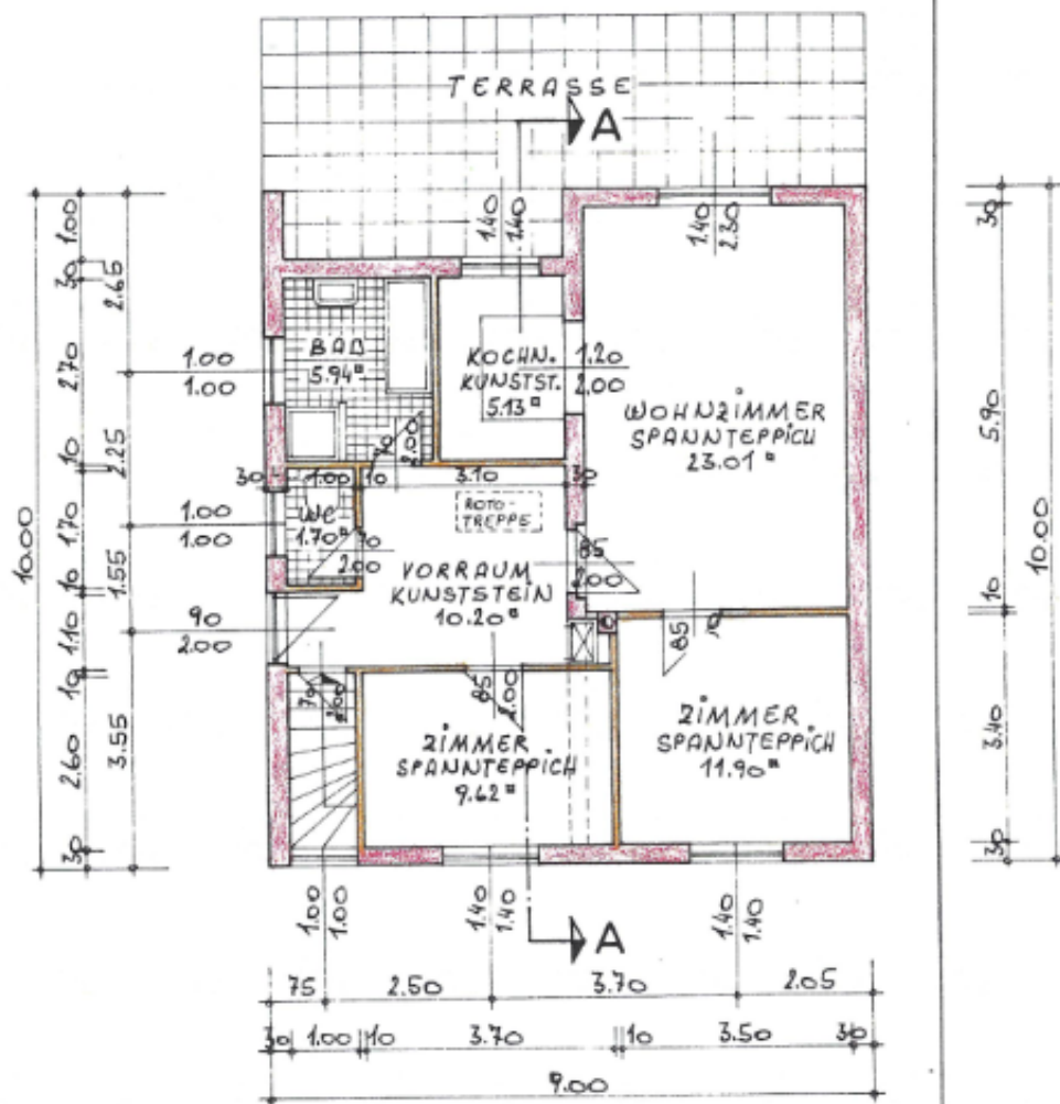
erdgeschoss 1:100
