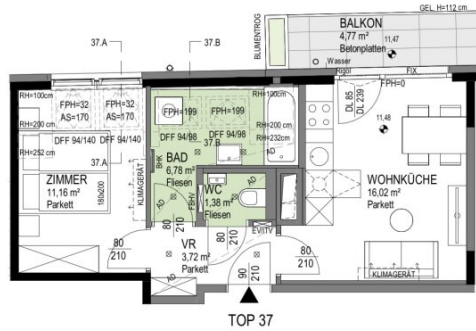
TOP 37
