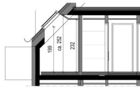
Schnitt 37.B
