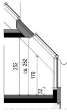
Schnitt 37.A
