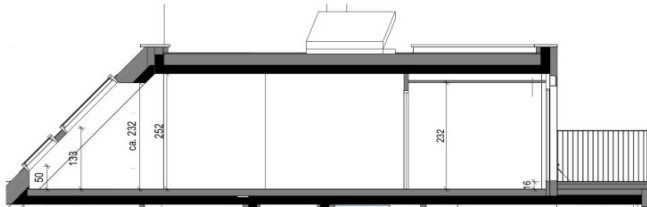
Schnitt 41.B
