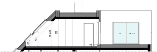
Schnitt 43.C
