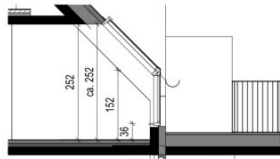
Schnitt 44.A
