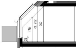
Schnitt 45.A
