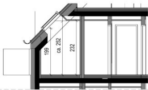
Schnitt 46.B
