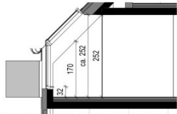
Schnitt 46.A
