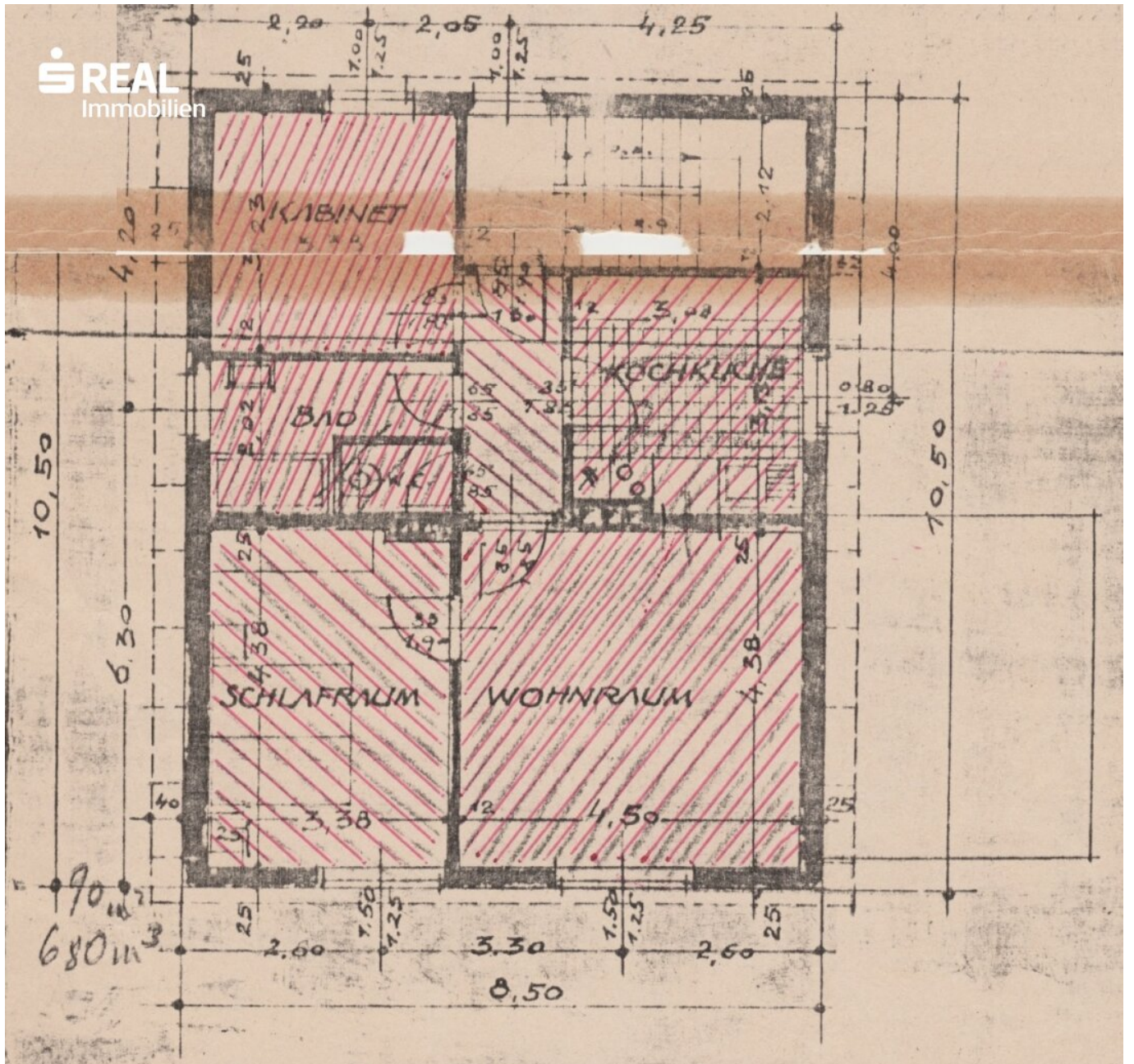
DACHGESCHOSSRUNDRISS
