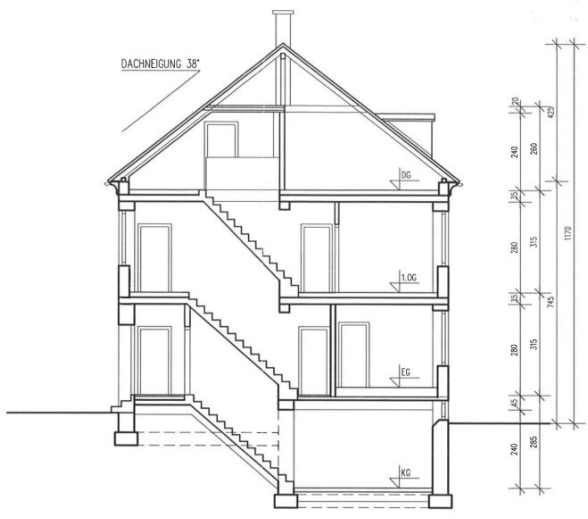
SCHNITT A-A
