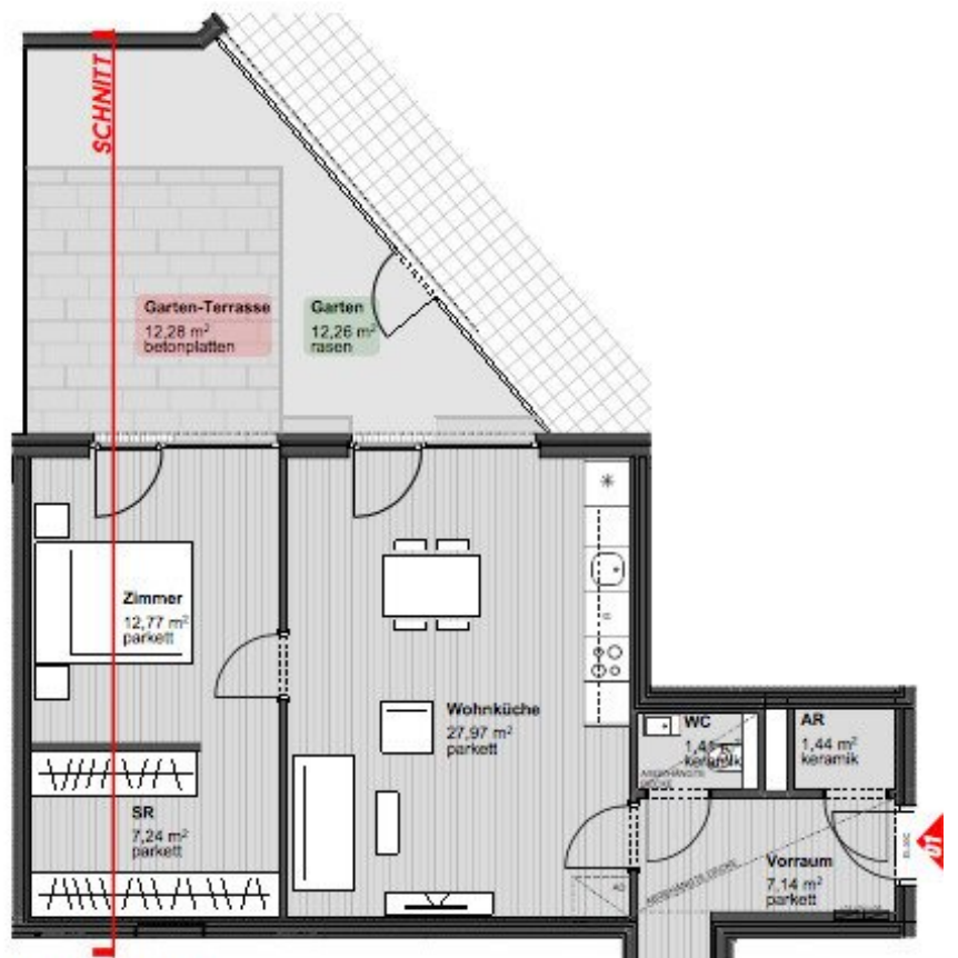
Grundriss | M 1:100
