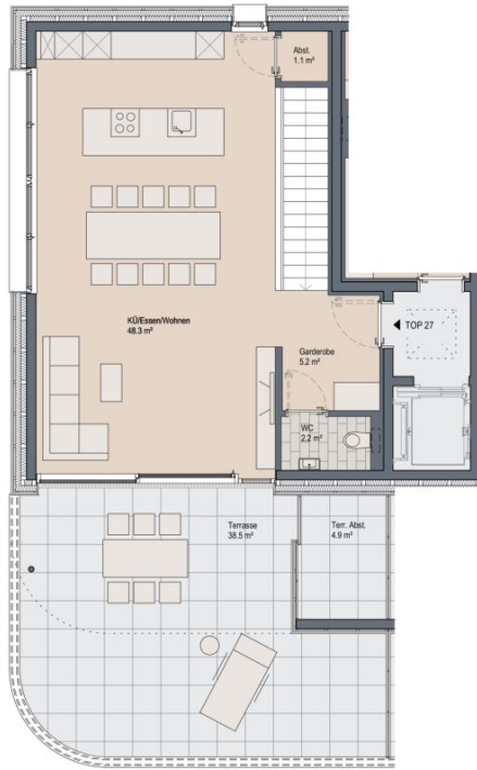
3. OBERGESCHOSS
