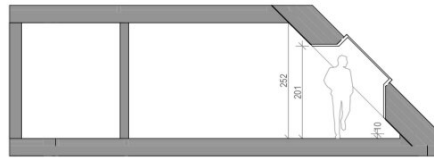
Schnitt 1-1
