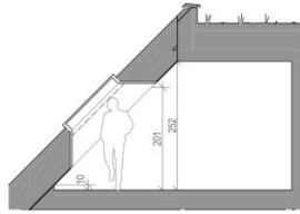
Schnitt 1-1
