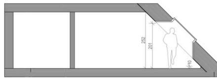
Schnitt 1-1
