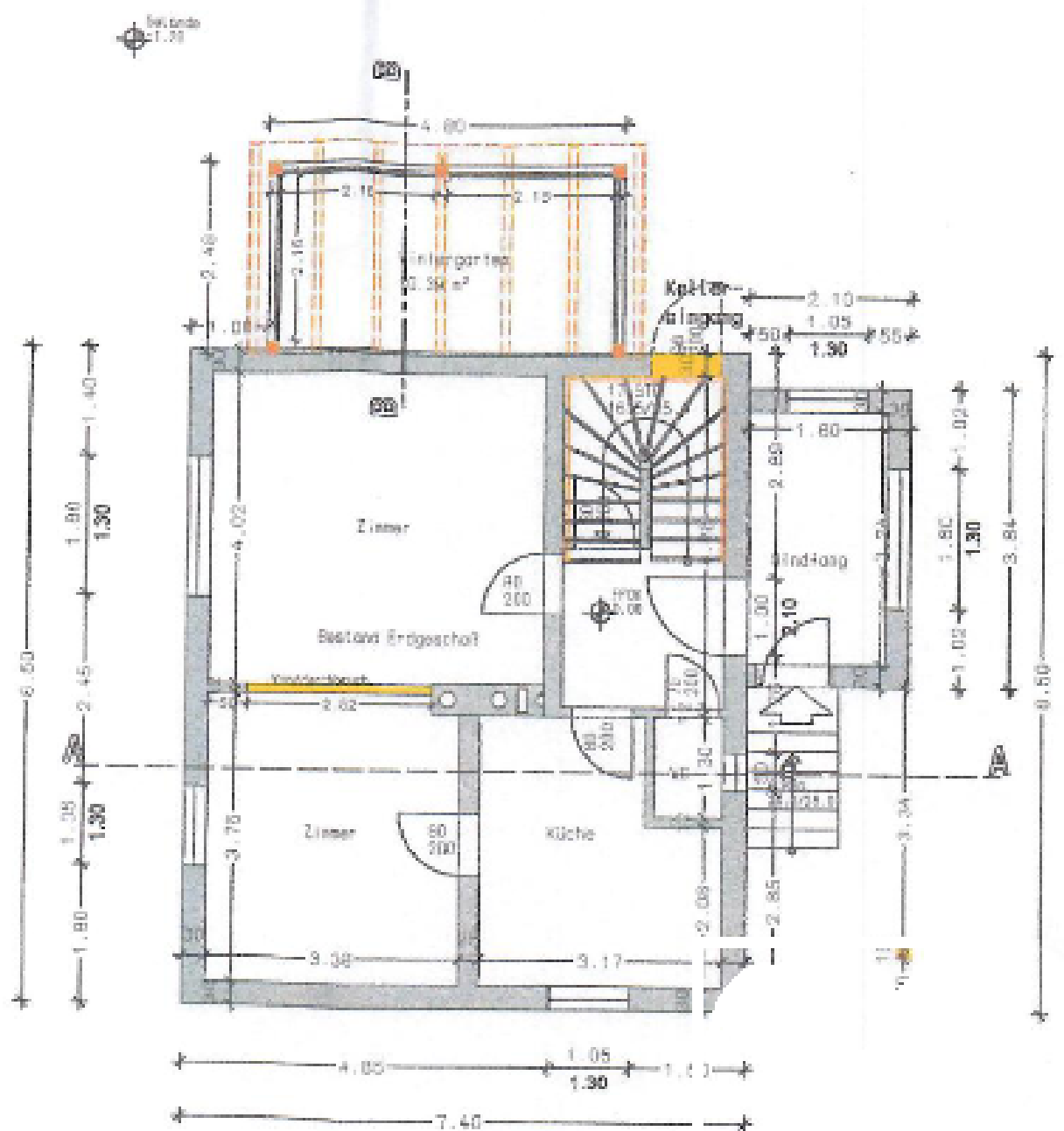
Erdgeschoss
