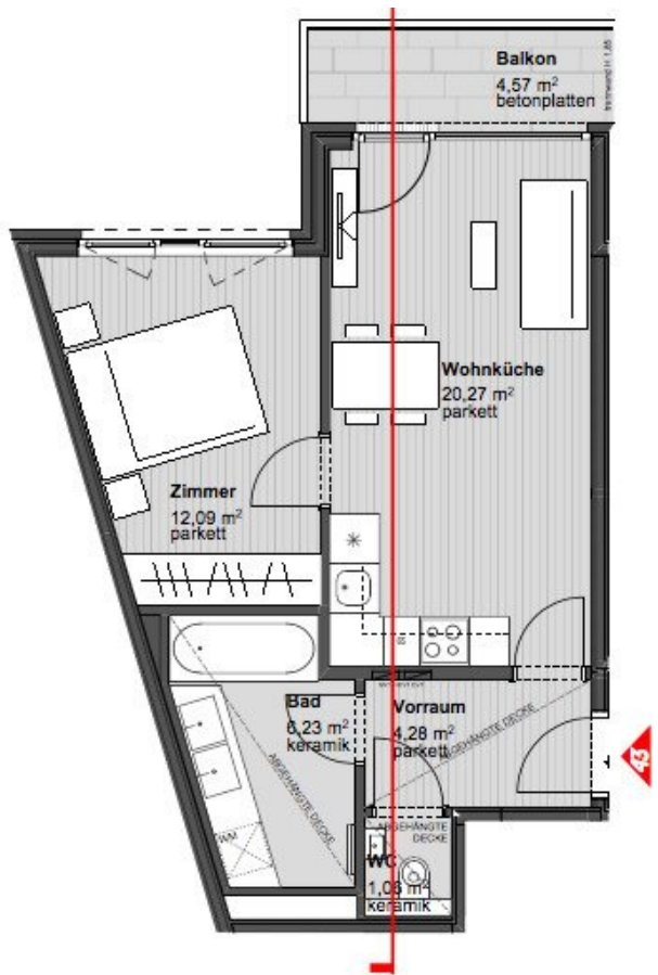
Grundriss | M 1:100
