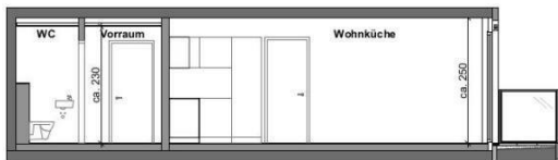
Schnitt | M 1:100
