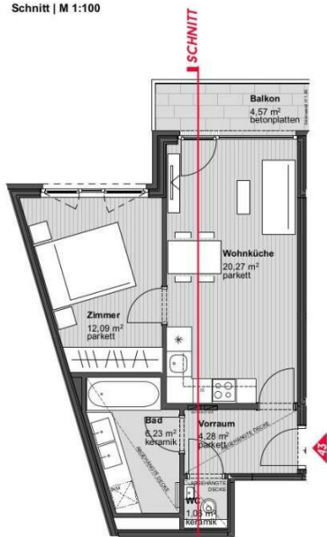
Grundriss | M 1:100
