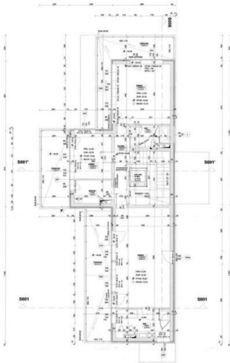
2. Obergeschoß
