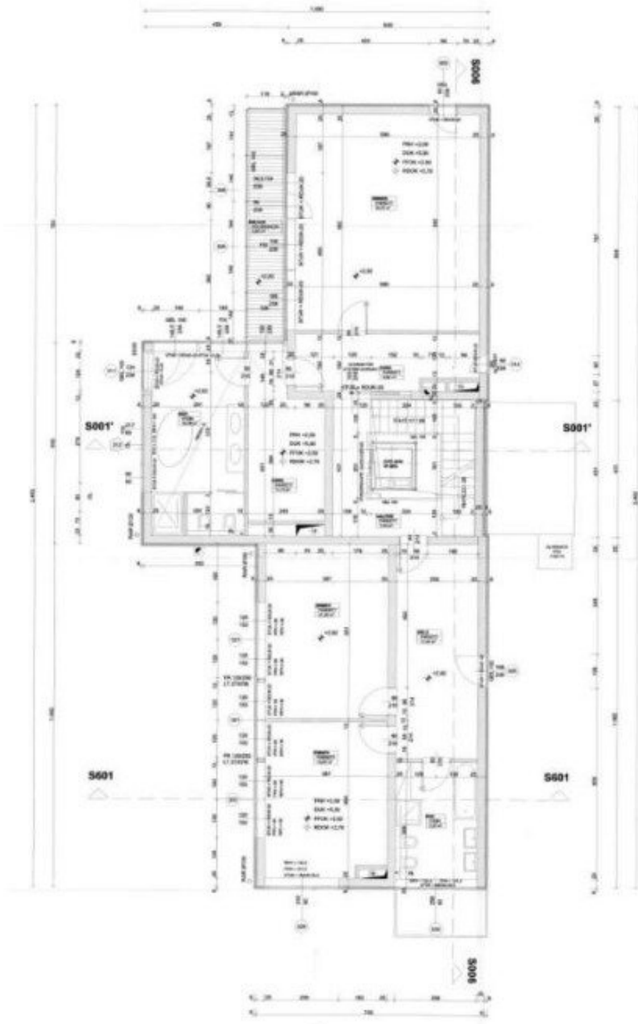
1. Obergeschoß
