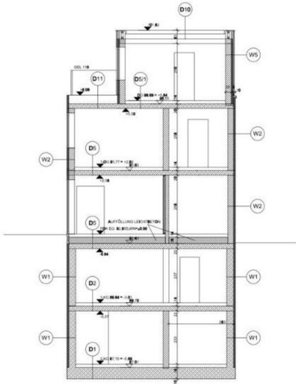
Relevante Höhenknoten innerhalb des Hauses
