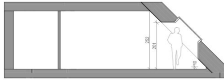
Schnitt 1-1
