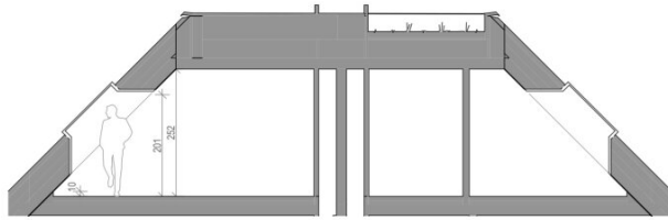
Schnitt 1-1
