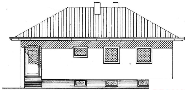
STRASSENANSICHT
