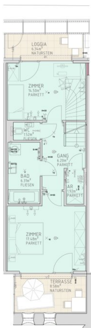
1.DACHGESCHOSS M 1:50
