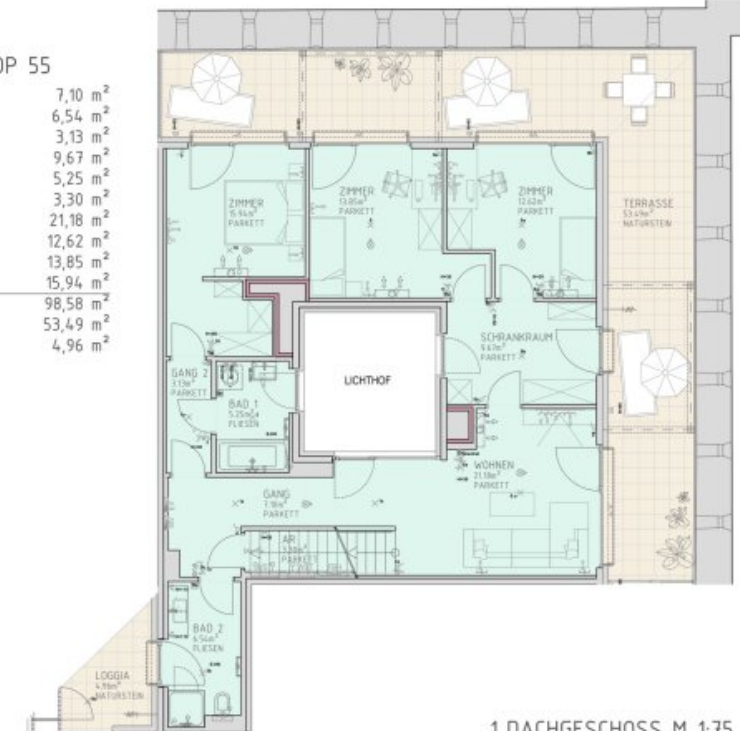
1.DACHGESCHOSS M 1:75
