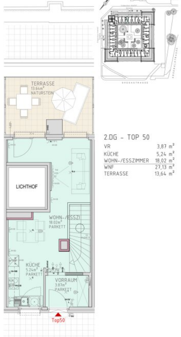
2.DACHGESCHOSS M 1:50
