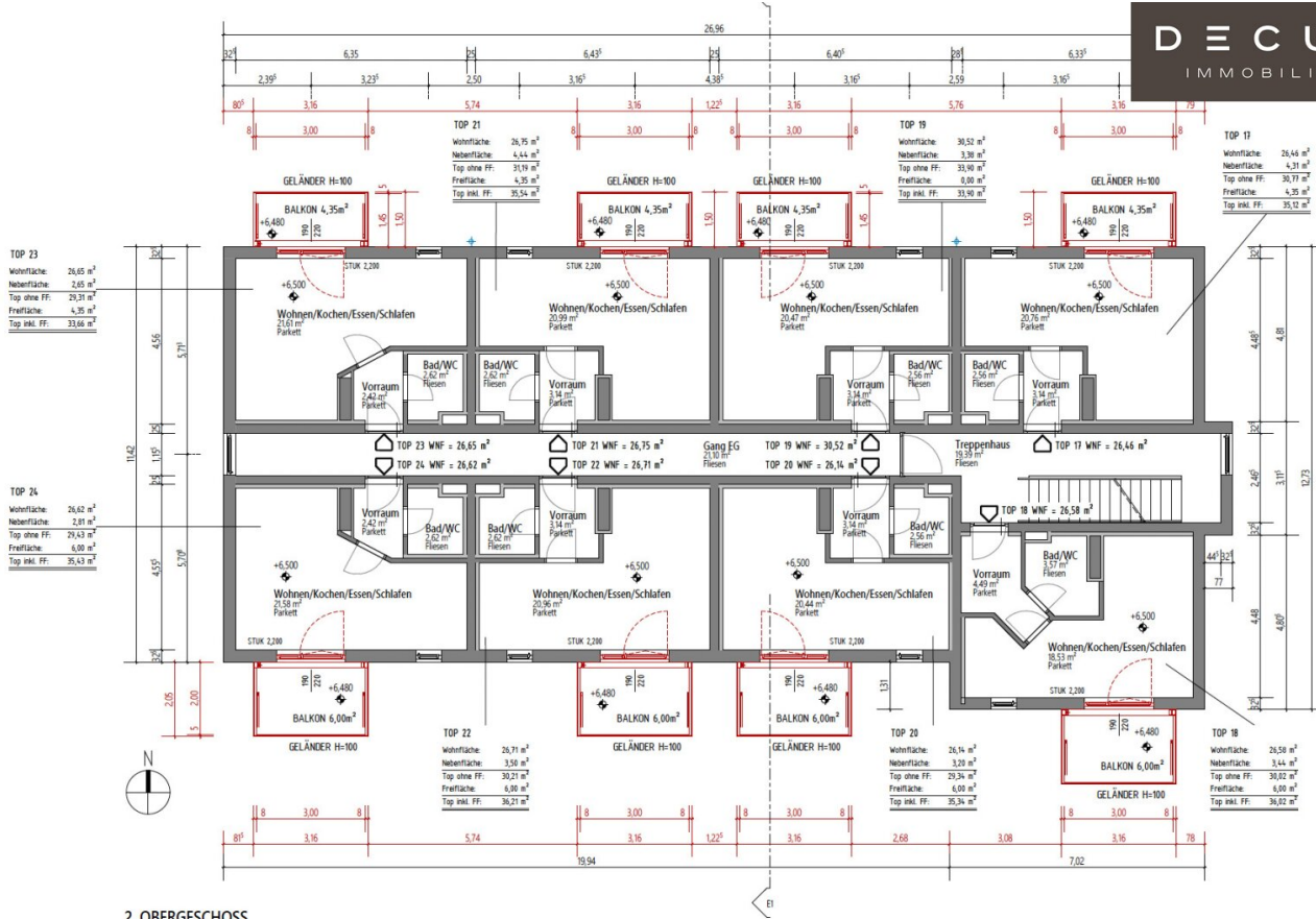
2. OBERGESCHOSS M 1:100
