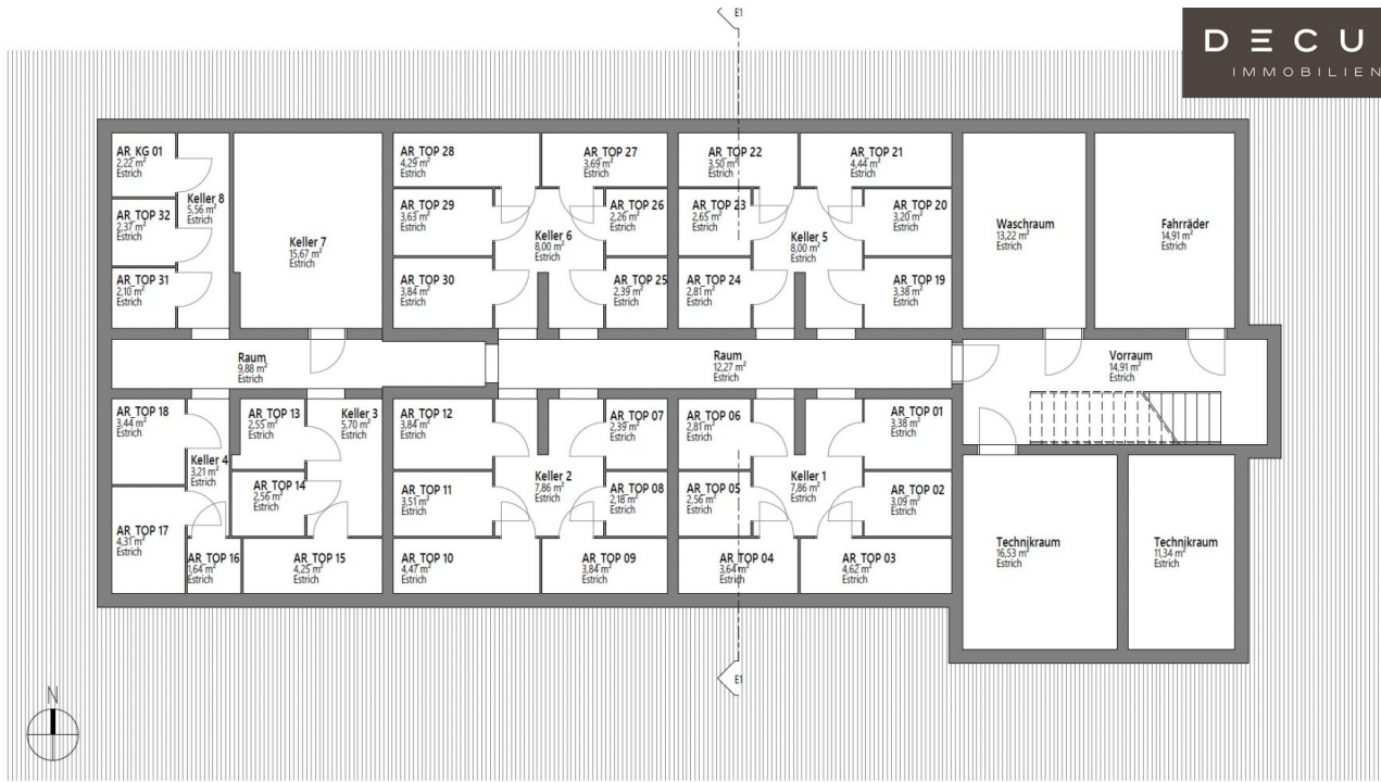
UNTERGESCHOSS M 1:100
