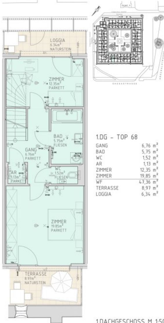
1.DACHGESCHOSS M 1:50
