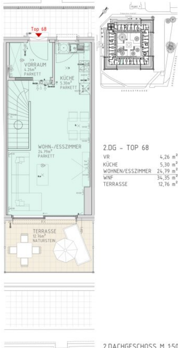
2.DACHGESCHOSS M 1:50
