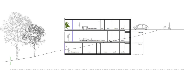
schnitt s1 - s1
