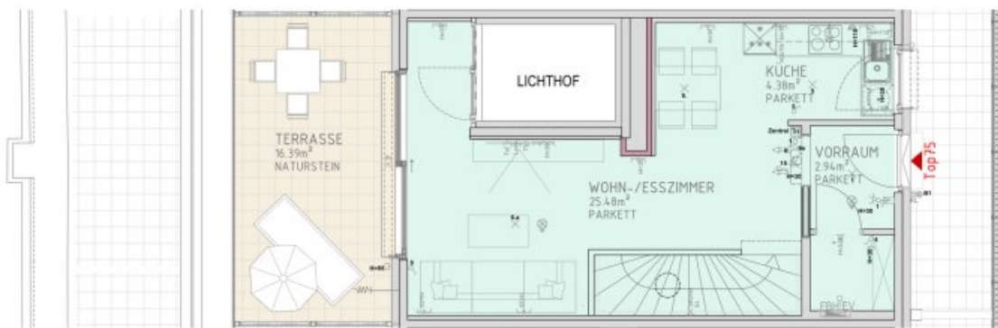
2.DACHGESCHOSS M 1:50
