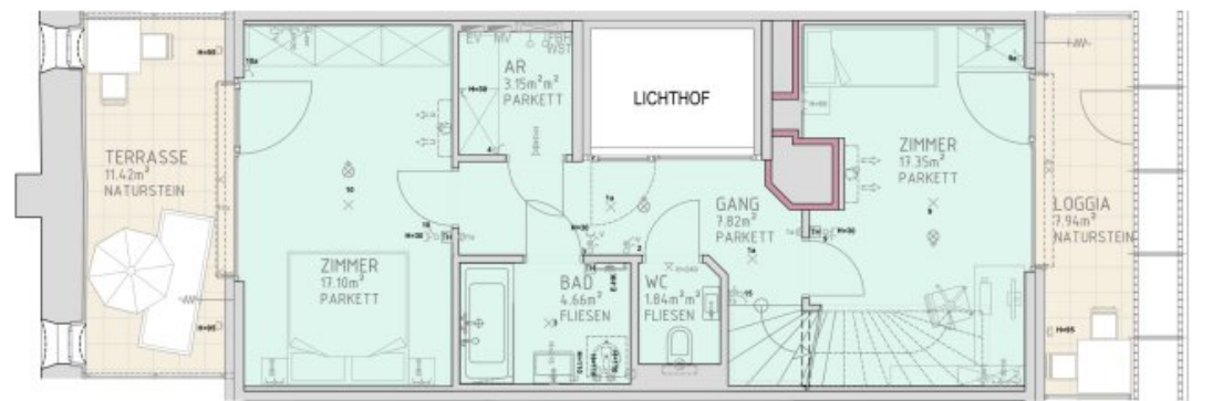
1.DACHGESCHOSS M 1:50
