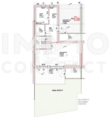
Reihenhausplan | Erdgeschoss RH 2
