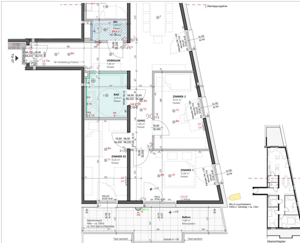
Übersichtsplan
