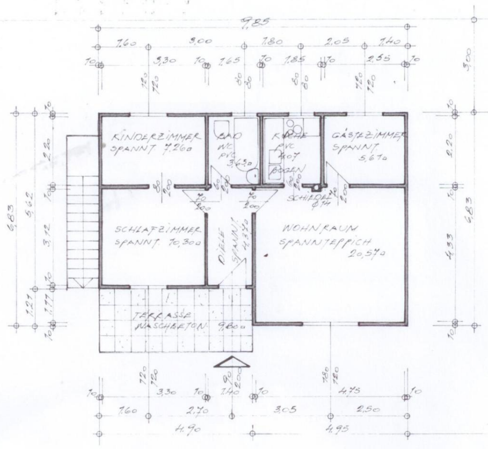
ERDGESCHOSS - GRUNDRISS
