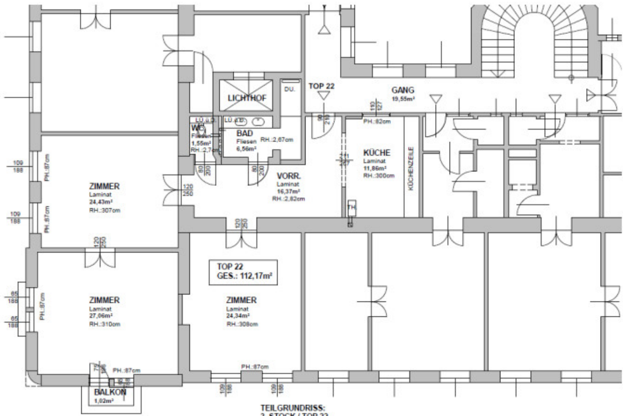
TEILGRUNDRISS: 3. STOCK / TOP 22
