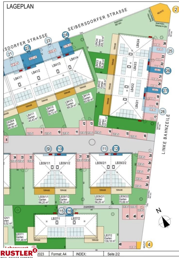
Lageplan 2
