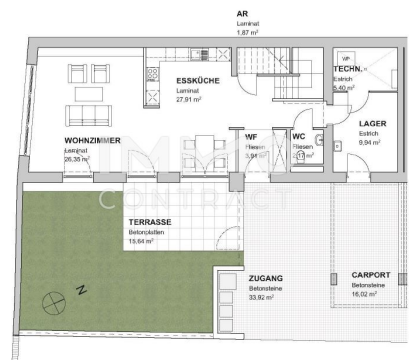
Reihenhausplan | Erdgeschoss RH 1
