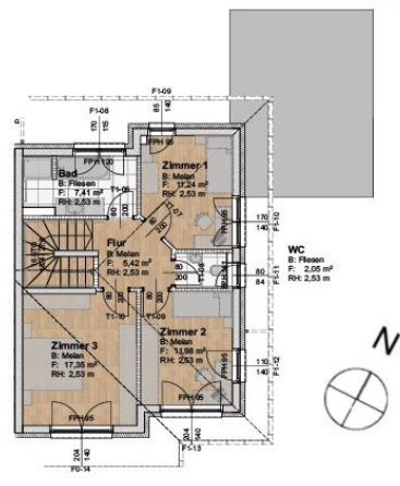
Reihenhausplan | RH.1, Obergeschoss
