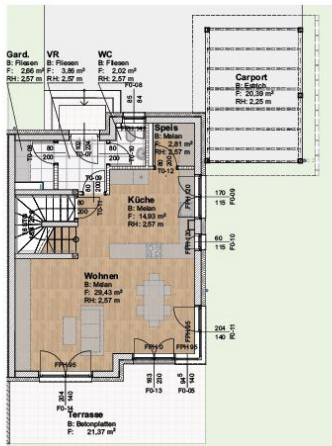
Reihenhausplan | RH.1, Erdgeschoss
