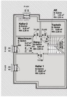
Reihenhausplan | RH 11, Kellergeschoss
