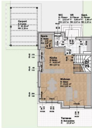
Reihenhausplan | RH 11 Erdgeschoss
