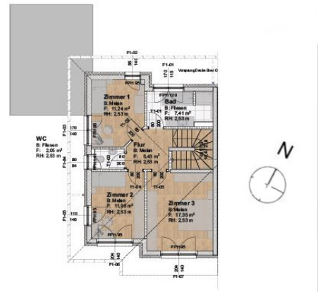
Reihenhausplan RH 11, Obergeschoss
