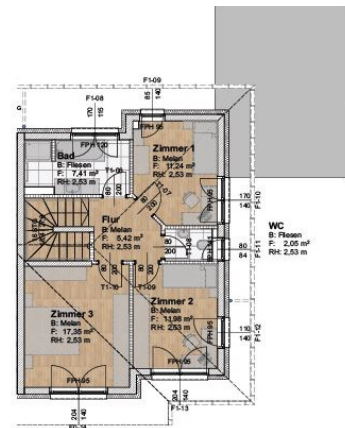
Reihenhausplan | RH 9, Obergeschoss
