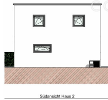
Südansicht Haus 2
