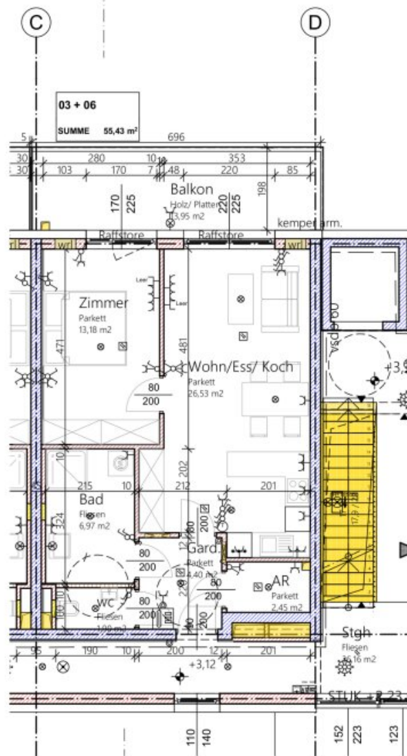
Obergeschoss
