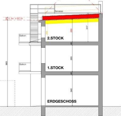
Schnitt Hoftrakt
