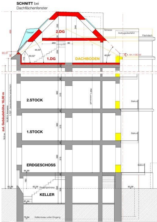
VORENTWURF
