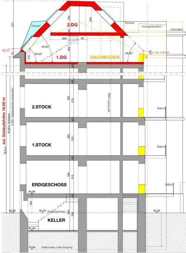
VORENTWURF
