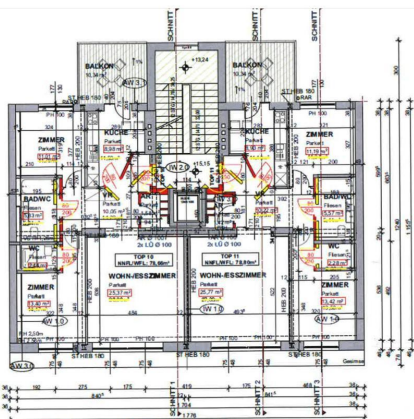
4. OBERGESCHOSS
