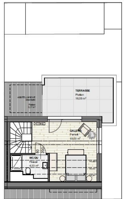
DACHGESCHOSS
