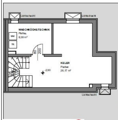
ÜBERSICHTSPLAN 1:250
