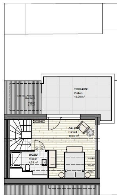
DACHGESCHOSS
