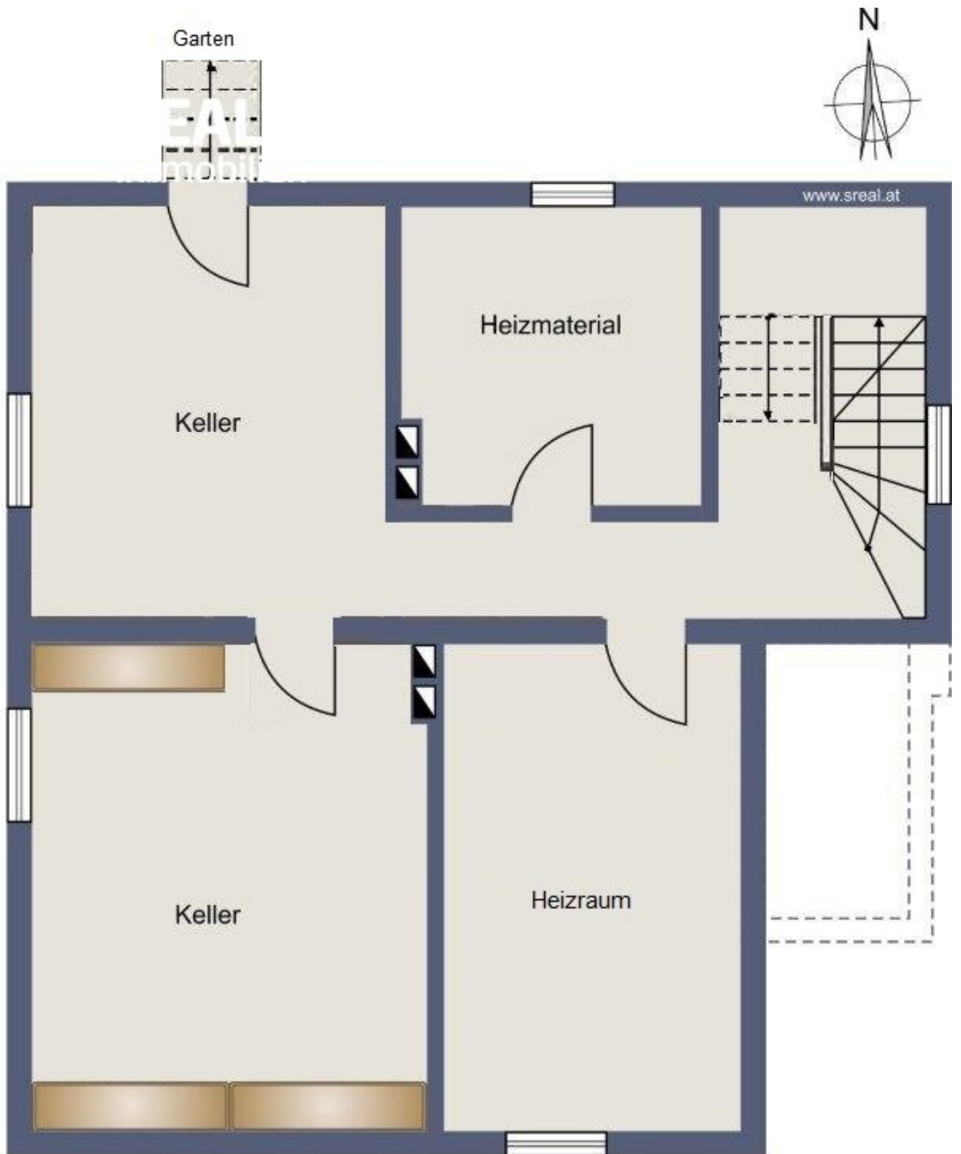
Skizze Kellergeschoss
