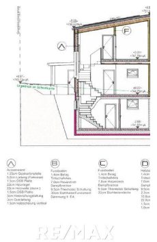
Haus: Schnitt
