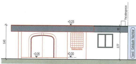
NORDWESTANSICHT
