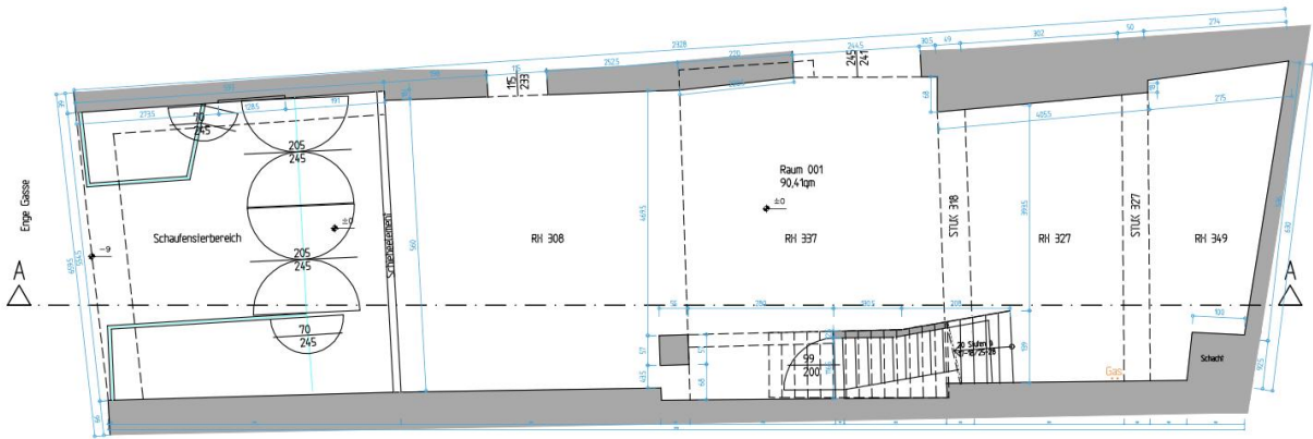
GRUNDRISS EG
