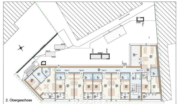
2. Obergeschoss
