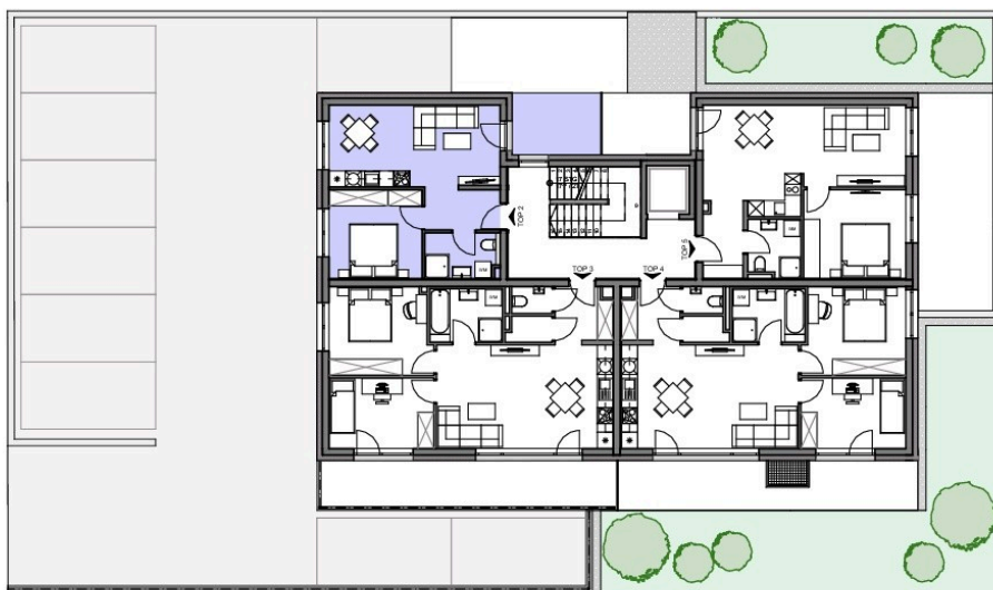
ÜBERSICHT 1.0G M=1:250
