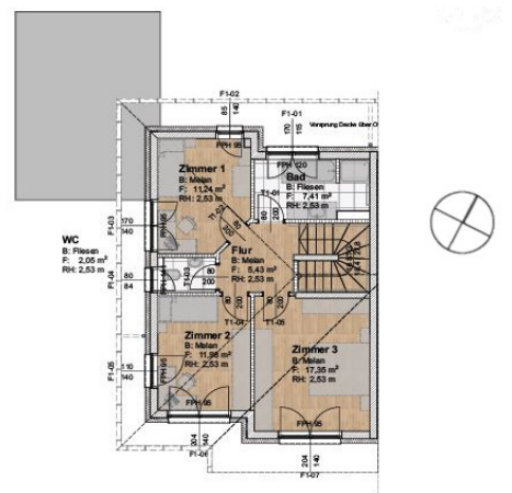
Reihenhausplan | RH3, Obergeschoss
