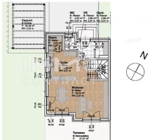
Reihenhausplan | RH 3, Erdgeschoss
