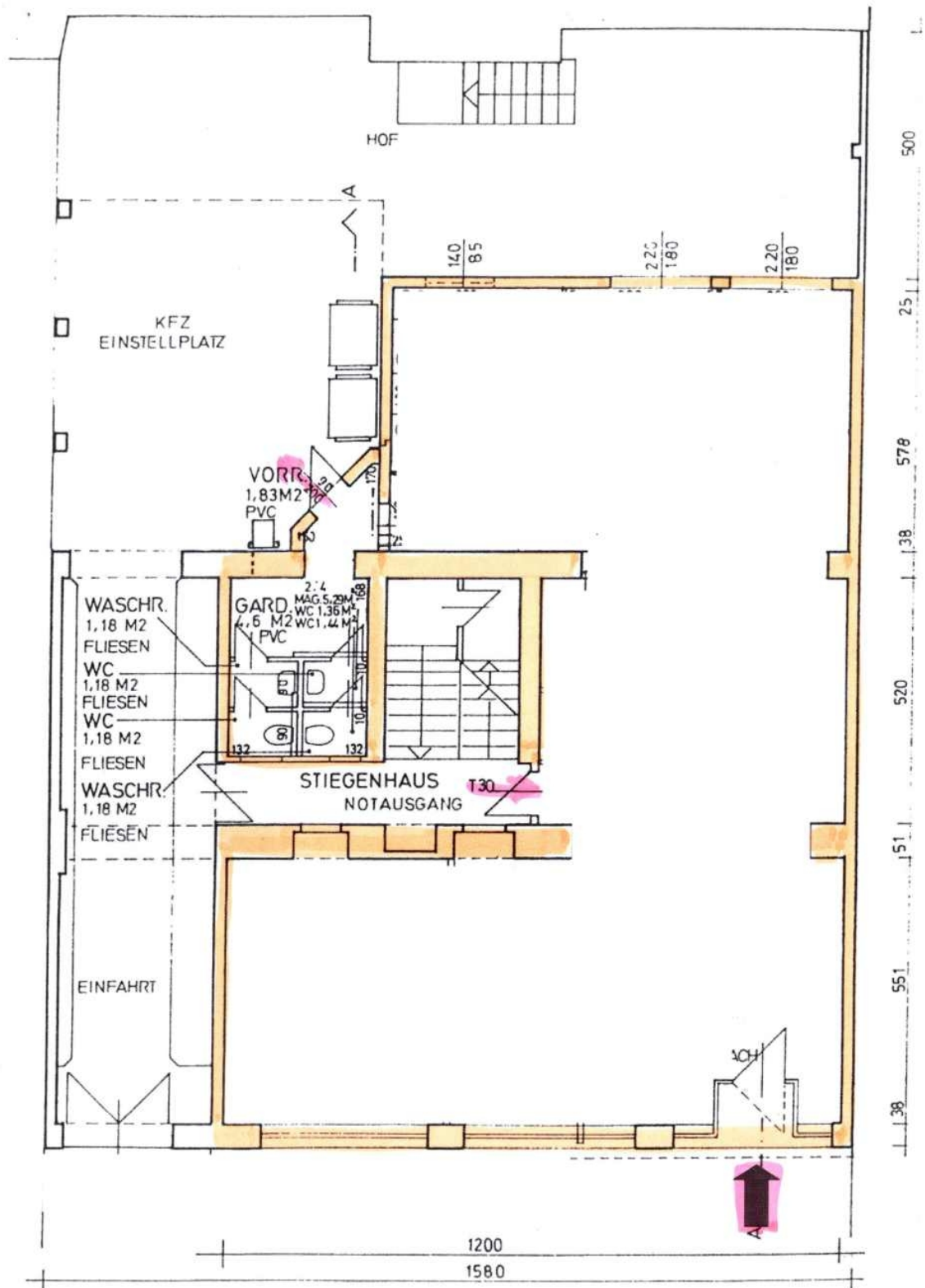
GRUNDRISS
