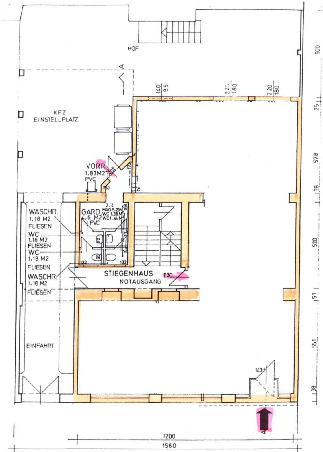
GRUNDRISS
